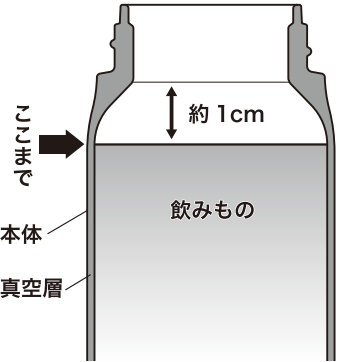
断面図
